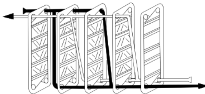
Figure 17. Plate heat exchanger (Lund, 1998).
