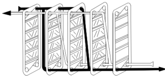
Figure 20. Plate heat exchanger (Lund, 1998).
